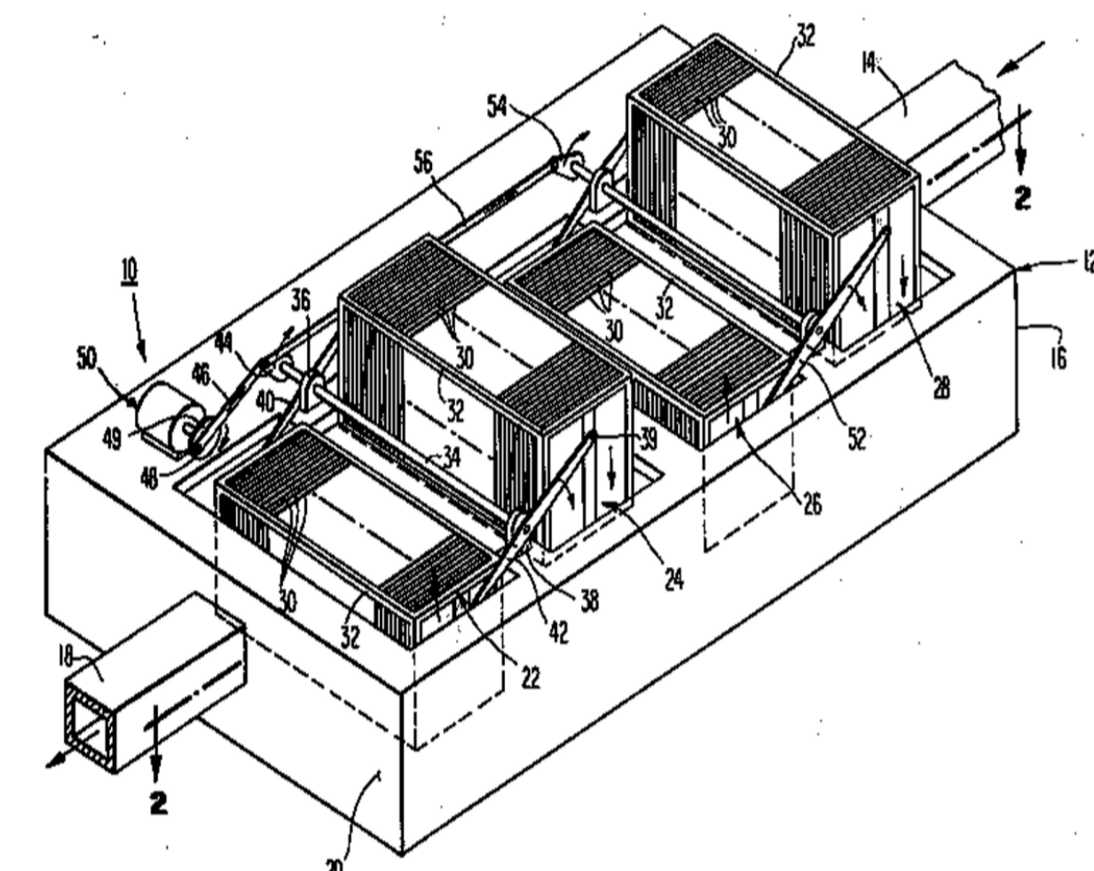
Abbildung 4: Entwurf aus einer US-Patentschrift mit einem Wipp-Antrieb. ROBERTS FILTER [1979]
