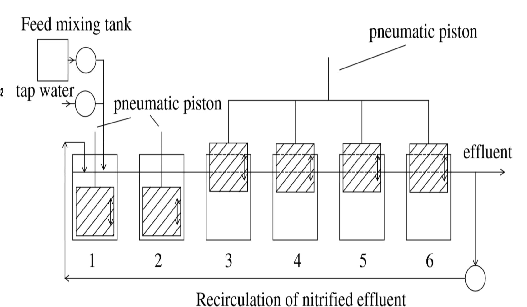
Abbildung 5: Darstellung eines kaskadierten Versuchsaufbaus zur Realisierung einer Stickstoffentfernung. RODGERS & BURKE [2003]
