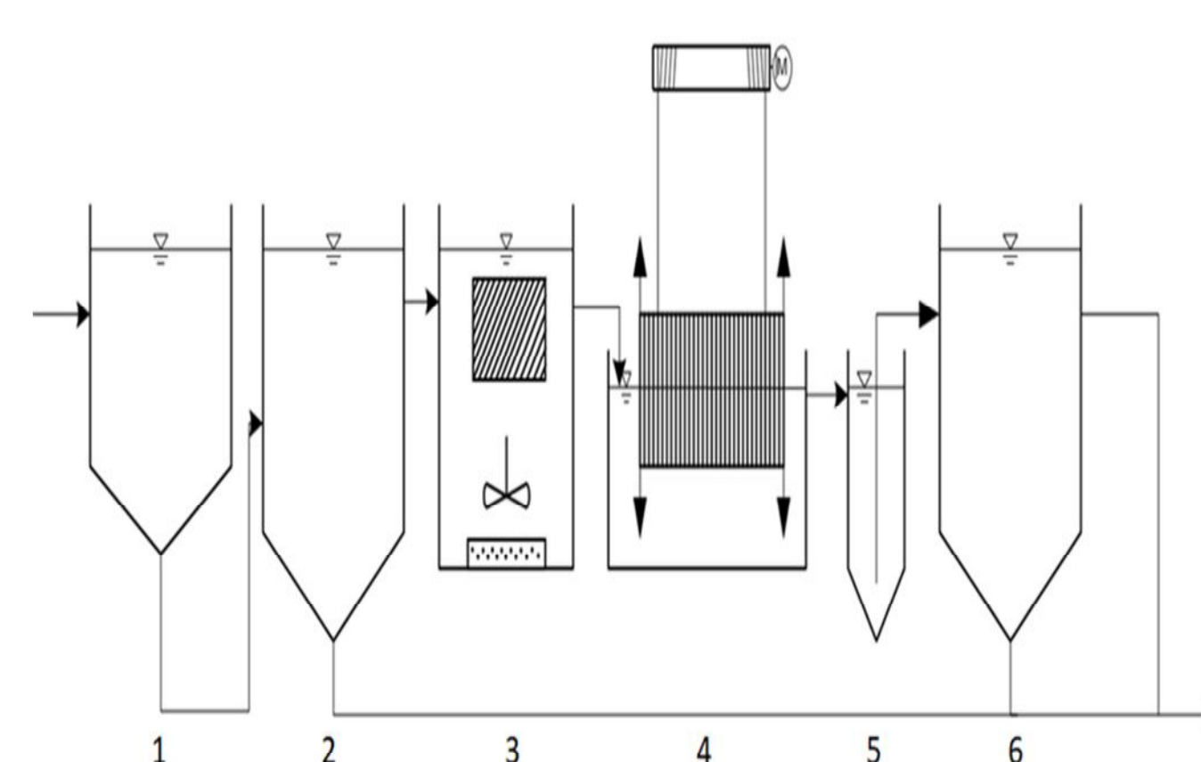
Abbildung 6: Schematische Darstellung des Versuchstandes an der Kläranlage Magdeburg, Gerwisch. (Bildquelle: CZOSKE)
