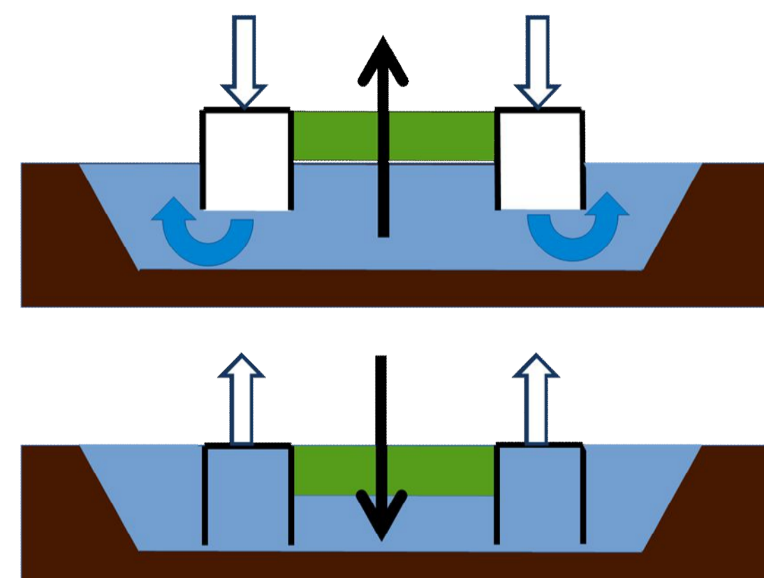
Abbildung 3: Aufgetauchte (oben) und getauchte (unten) Position. CZOSKE [2016]
