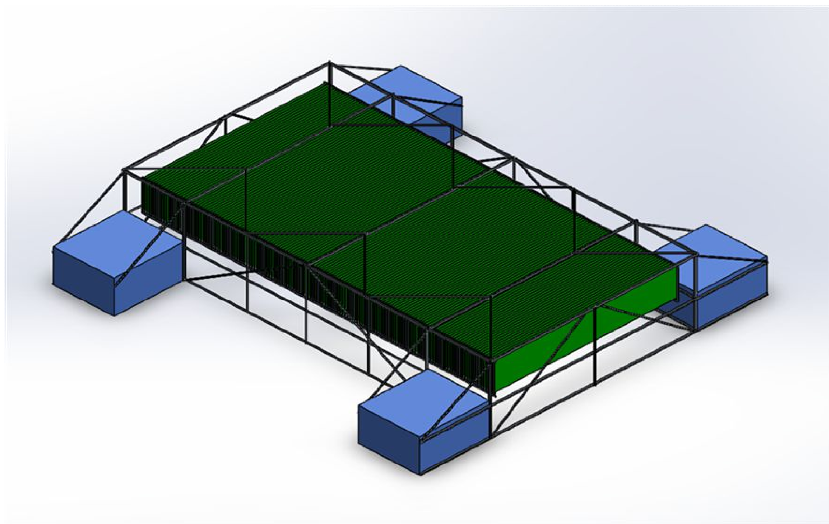
Abbildung 1: Isometrische Darstellung eines Schwimmtauchkörper-Prototyps mit seitlich angebrachten Tauchglocken (blau) und innen gespannte Folien oder Netze als Aufwuchsflächen (grün). CZOSKE [2016]
